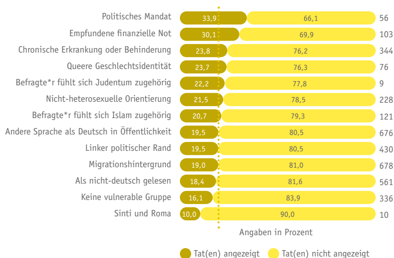
Abbildung 4: Gruppenspezifisches Anzeigeverhalten (gelbe Linie markiert die durchschnittliche Anzeigequote)
