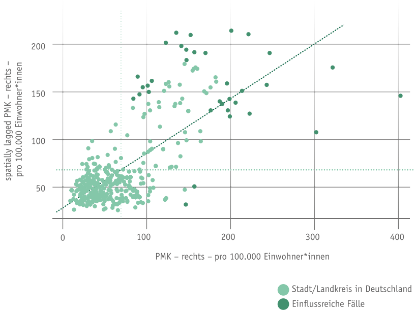
Abbildung 4: Moran's I Scatterplot von politisch rechtsmotivierten Straftaten in Kreisen pro 100 Tsd. Einwohner*innen im Jahr 2022 (Grafik erstellt mit dem spdep Paket in R)
